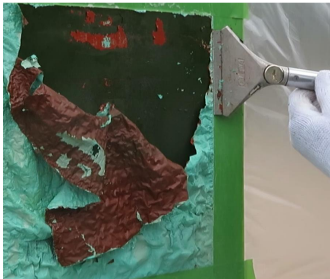
剥離剤塗布後 塗膜を剥離する様子
