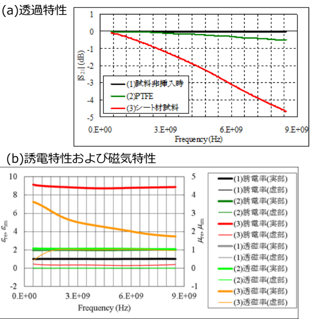
図1. 同軸管法による各種特性 (2ポート測定系)
