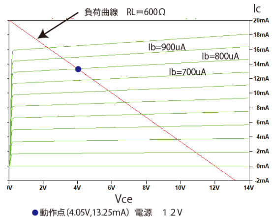
図1 2SC1815の動作曲線
