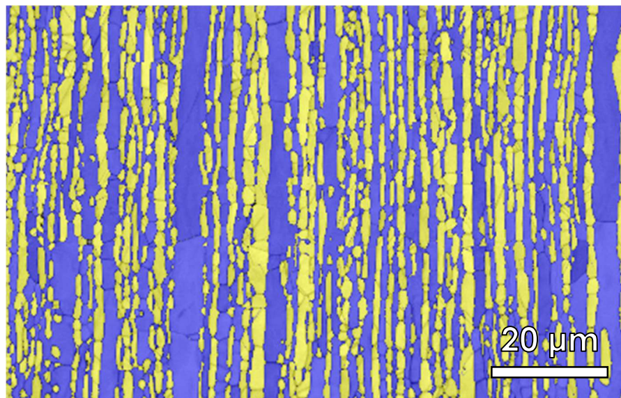
二相ステンレス鋼(SUS329J4L)のフェーズマップ
